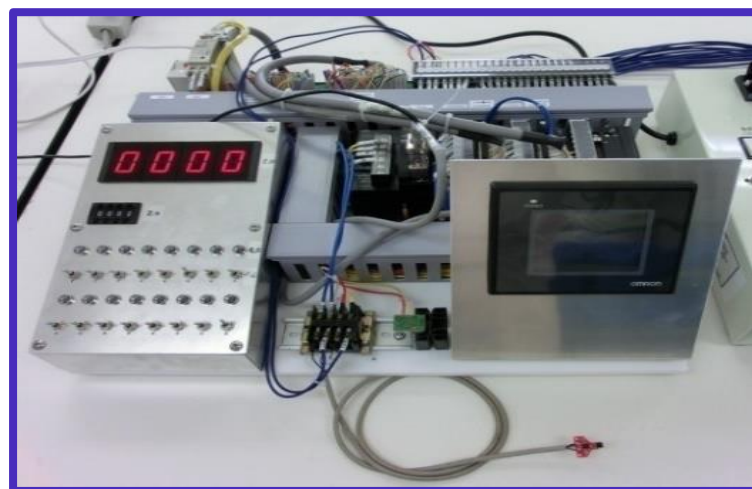
〔実習P L C機材(オムロン)〕
