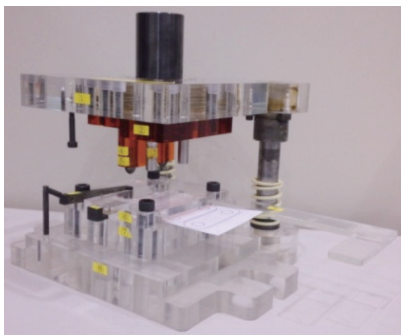
アクリル製プレス金型モデル
