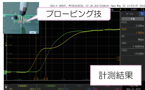
回路計測の一例
