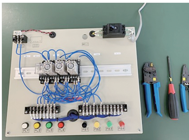
(制御盤用教材の例)
