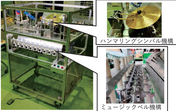
令和2年度専門課程総合制作実習 最優秀賞受賞 【メカニカルオーケストリオン製作】
