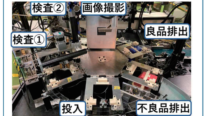
令和3年度応用課程開発課題実習 最優秀賞受賞 【溶接ボルトスパッタ自動判別装置の開発】
