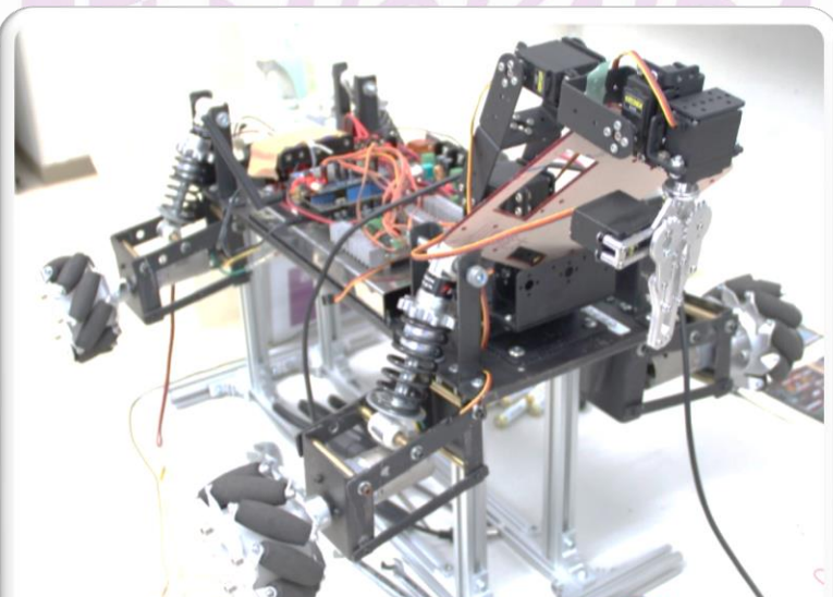
全方向移動可能アームロボット
