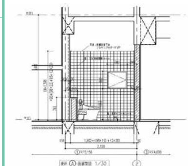
タイル割付図(展開図)
