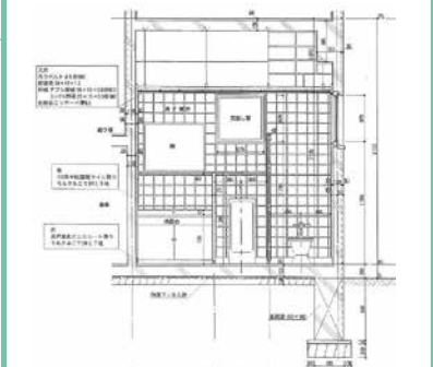
タイル割付図(展開図)
