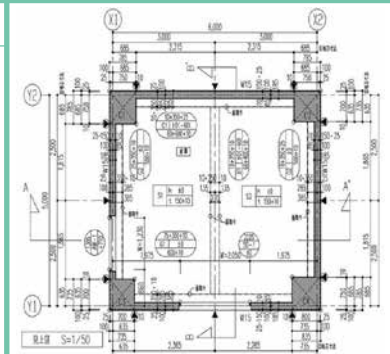
見上げ平面図
