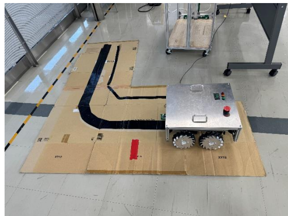
牽引型AGVの制作
