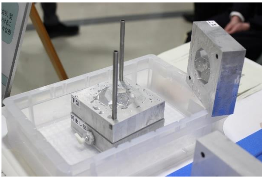
小型放電加工機的设计・製作
