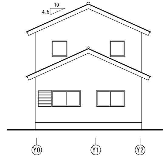
東立面図
