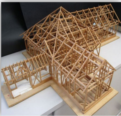
木造住宅の架構
