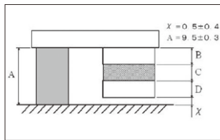
寸法公差の考え方
