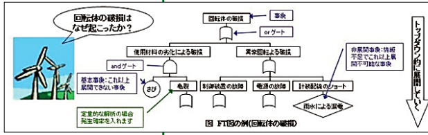
FTA図の例
