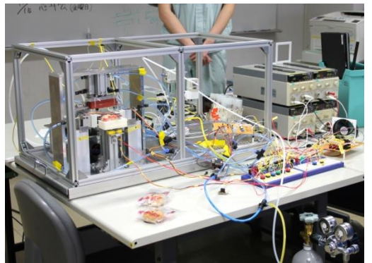
企業との共同研究「酸素除去包装装置」の開発室にて
