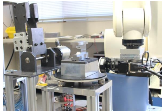
企業との共同研究「三次元検査システム装置」の開発室にて
