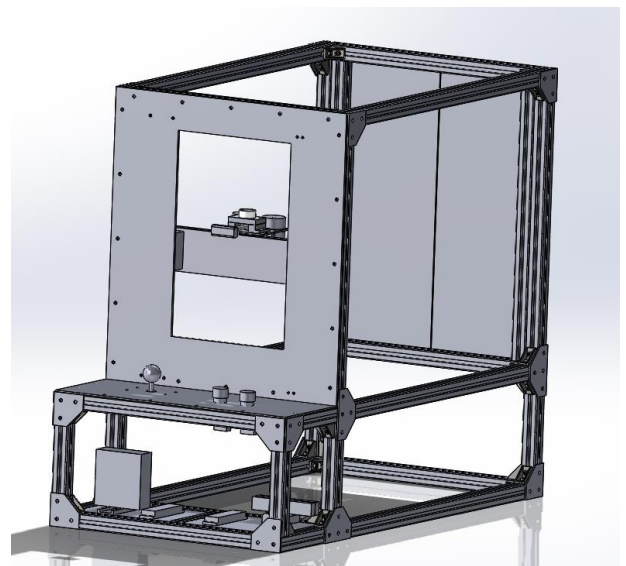
図3 全体のモデリング
