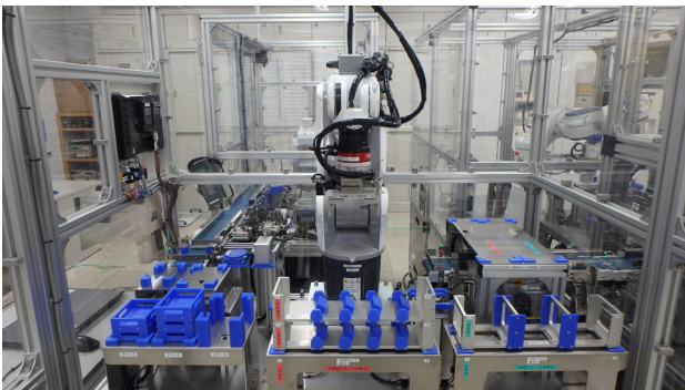
図6 基板組立仕分けステーション
