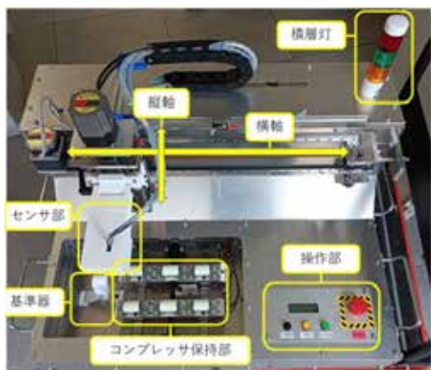
図 15 全体外観(前面)
