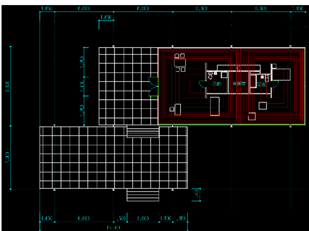
図12 床暖房配線図
