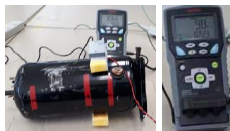
図 11 LCR メータ「LCR700」の基礎実験
