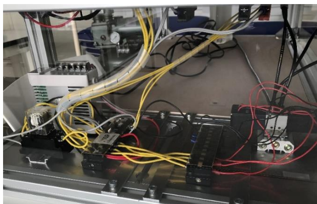
図8 線の長さを調整した配線
