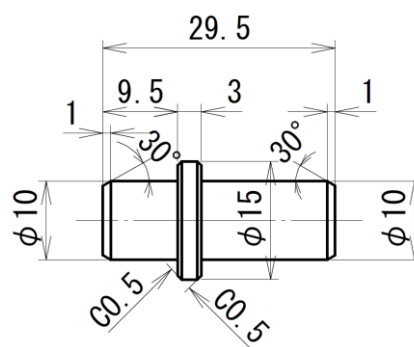
図11 ワークの形状
