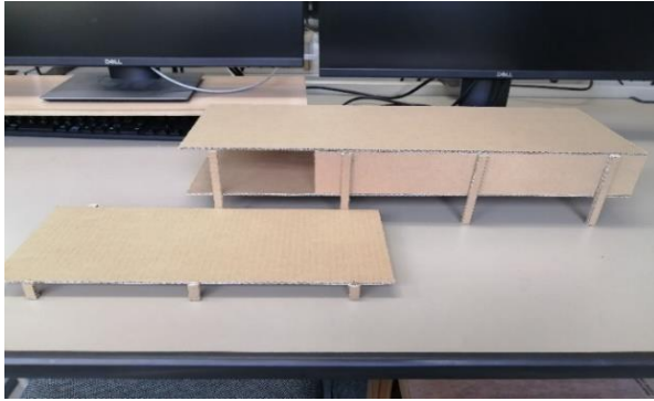
図5 ダンボール試作模型 (S=1/50)
