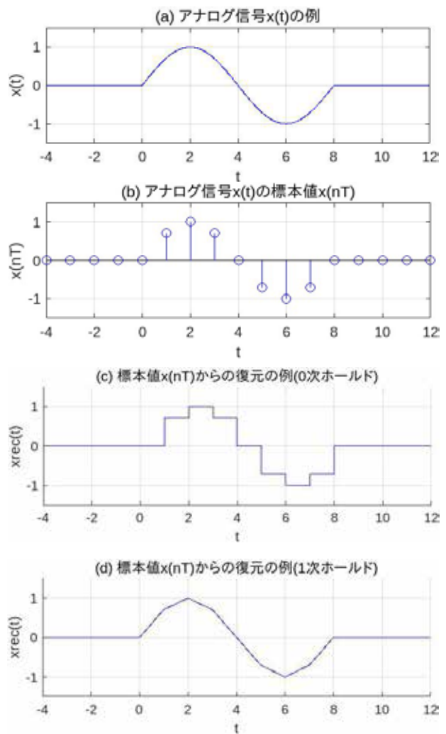
図1 アナログ信号の標本化と復元の例
