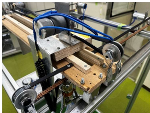
図 1 改良した動作部
