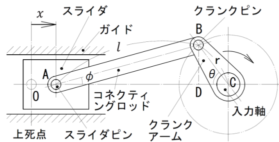
図7 クランク軸角変位 \theta スライダ位置 x の関係
