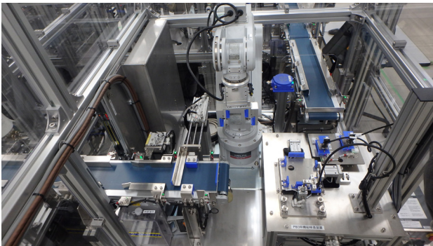
図5 基板検査ステーション
