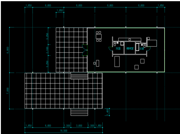
図11 平面図機械室扉位置
