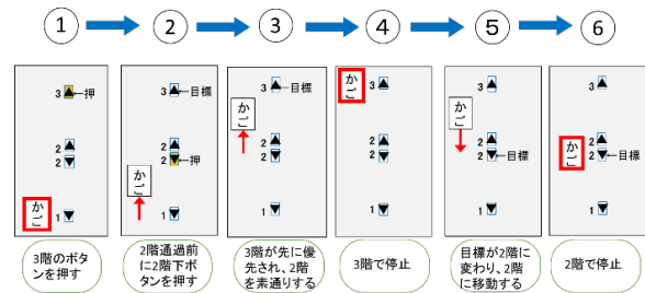
図7 動作例2
