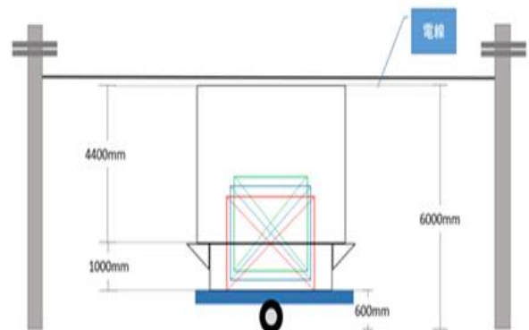
図2 概要図(格納時)
