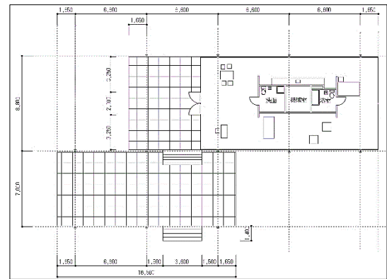
図1 平面図(S=1/100)
