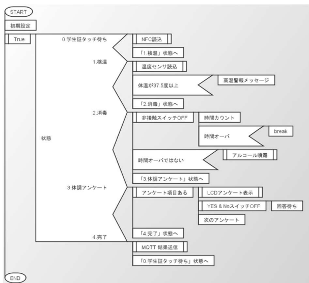
図5 端末制御プログラム
