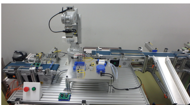
図10 基板検査装置
