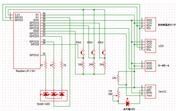
図4 インタフェース回路
