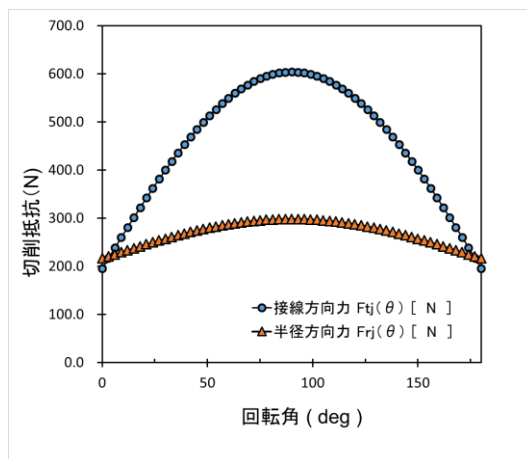
図2 切削抵抗
