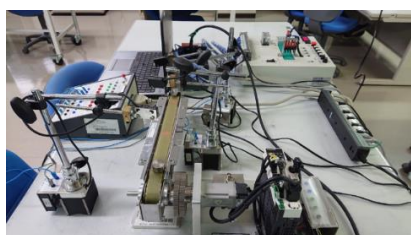
図1 プログラム作成用模擬装置
