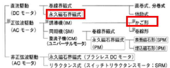
図 2 モータ分類
