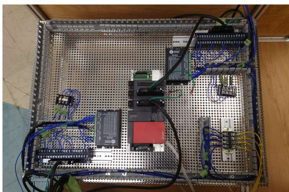
図 5 制御部
