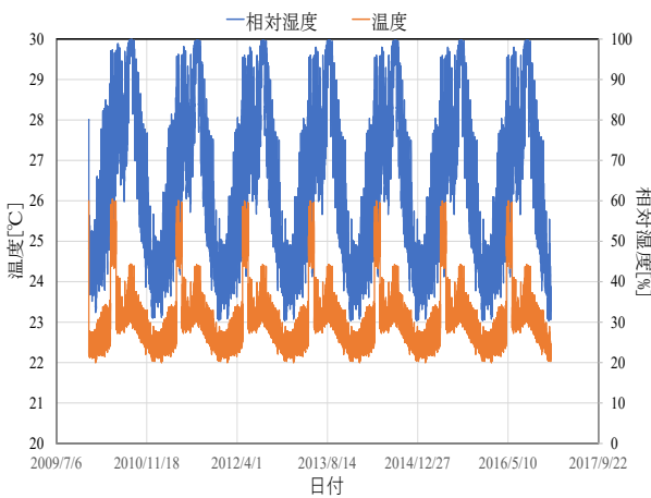
図 12 GW—石膏ボード間の温度・湿度の計算結果
