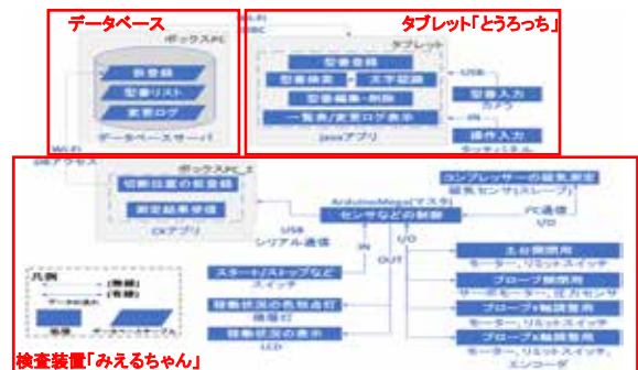
図5 システムの全体構成図
