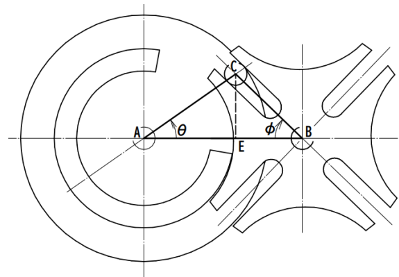
図 2 入力軸角変位 \theta における原動ホイールと被動ホイールの姿勢
